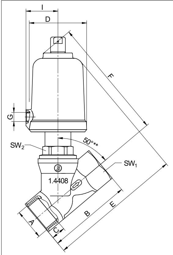
Feder schließt
