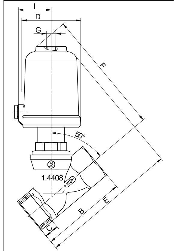
Feder öffnet
